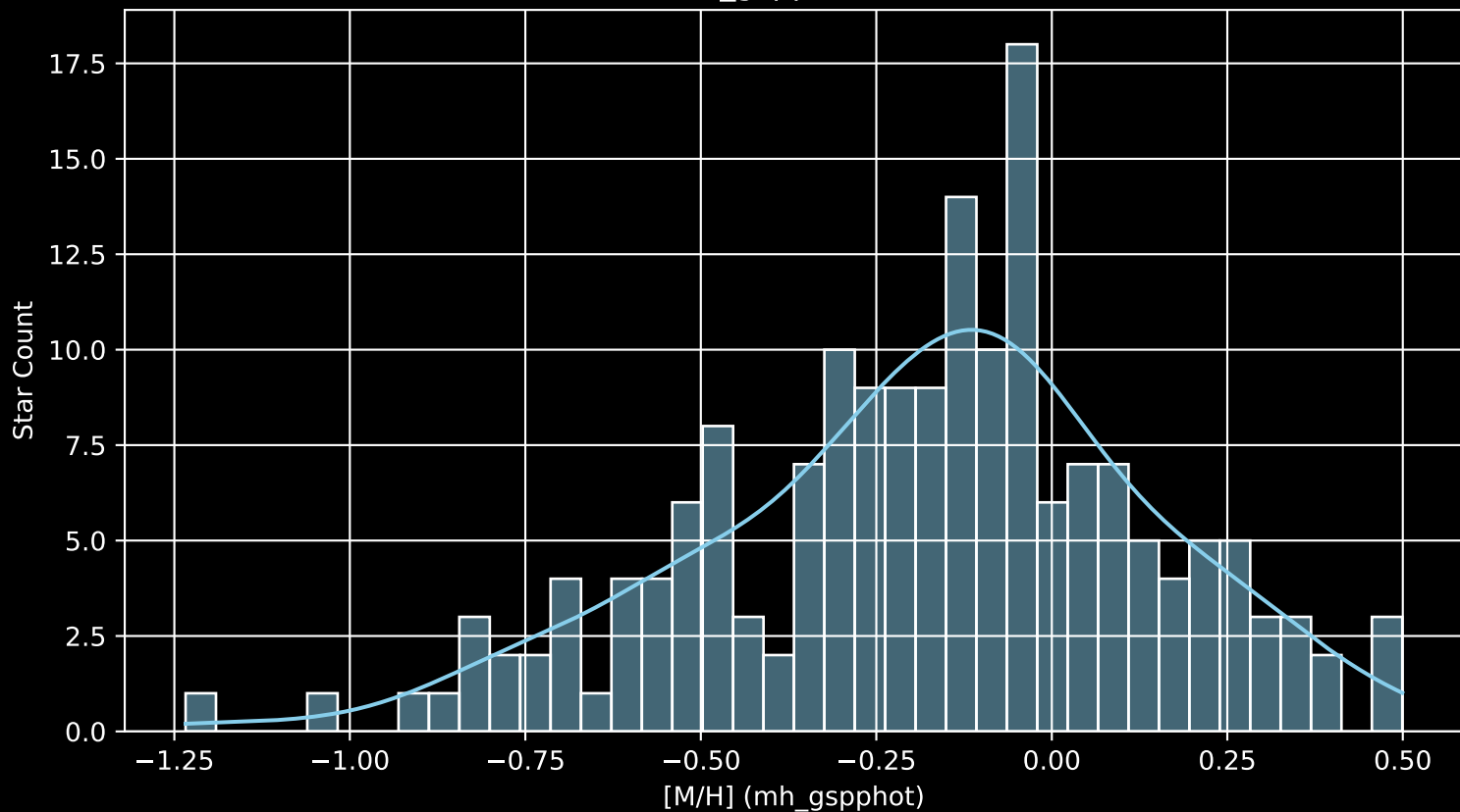
APOGEE DR17 Field: [151+60 MGA [M/H] (mh_gspphot) (n= 179)
