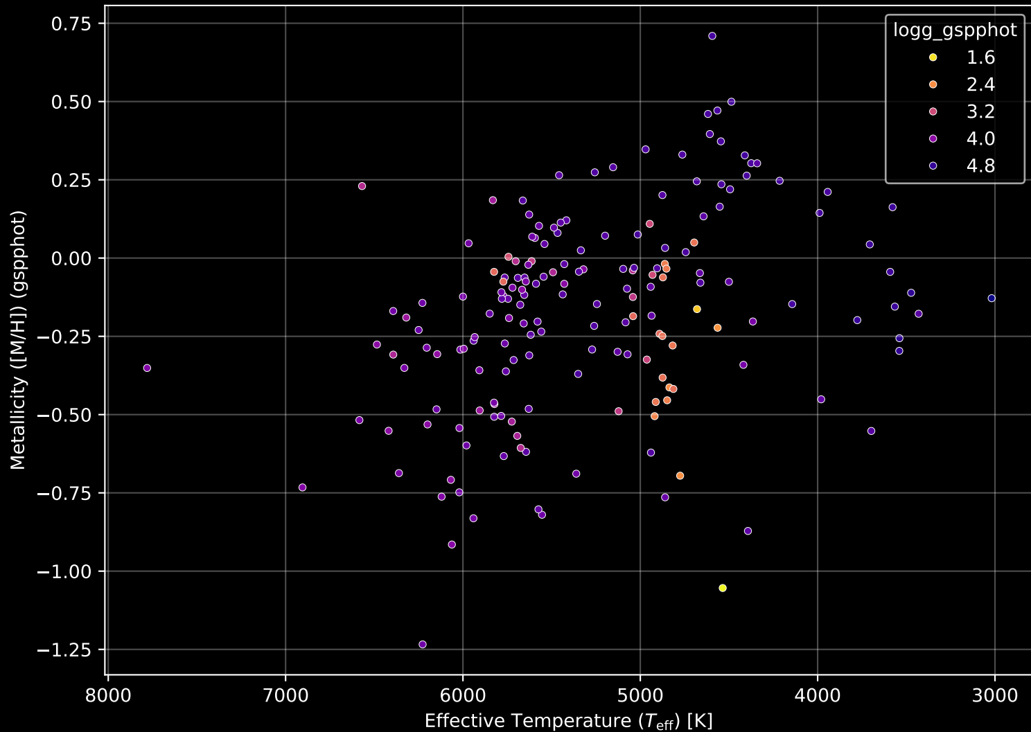
APOGEE DR17 Field: [151+60_MGA] Stellar Population Parameters (n= 180)
